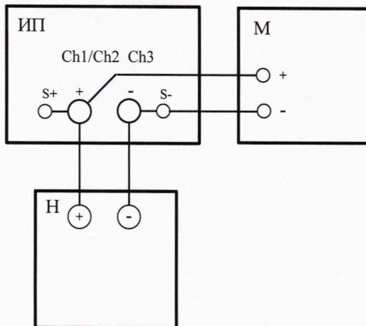
Рисунок 1 – Схема подключения оборудования при определении абсолютной погрешности воспроизведения напряжения постоянного тока, где ИП – источник питания Rigol DP2031;
